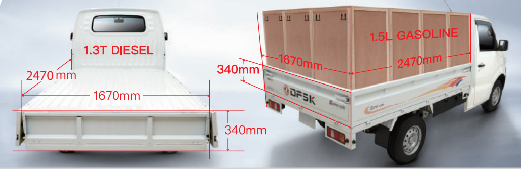
4-strip Cubical Support Rack dengan 16 buah Cargo Bed Reinforcement Bars agar lebih tahan lama
