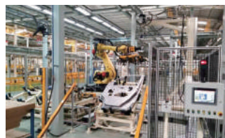
Area Pengelasan
